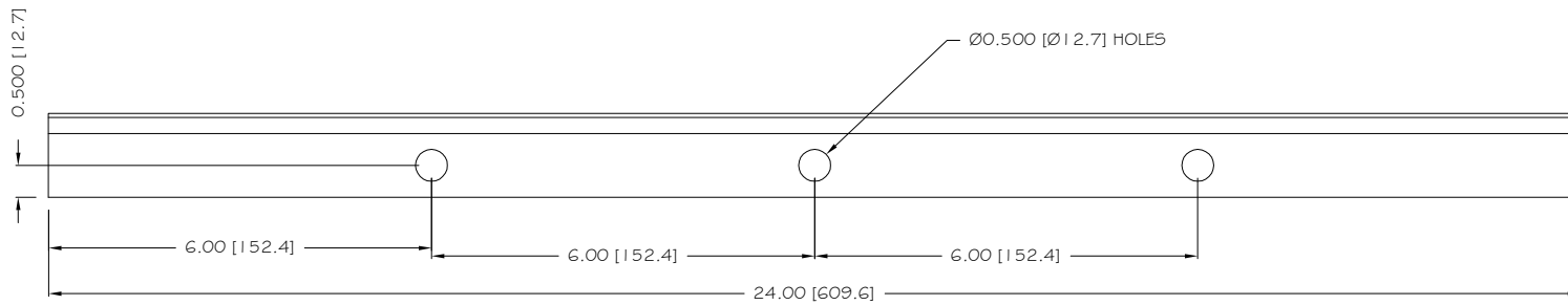
SECTION A-A
